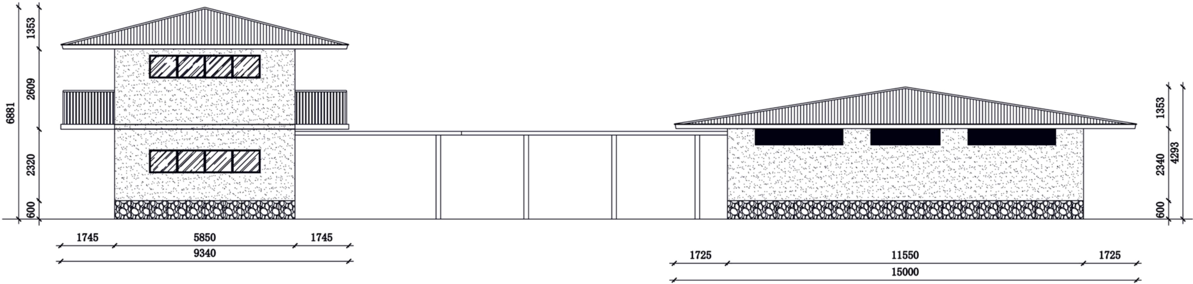
立面图
