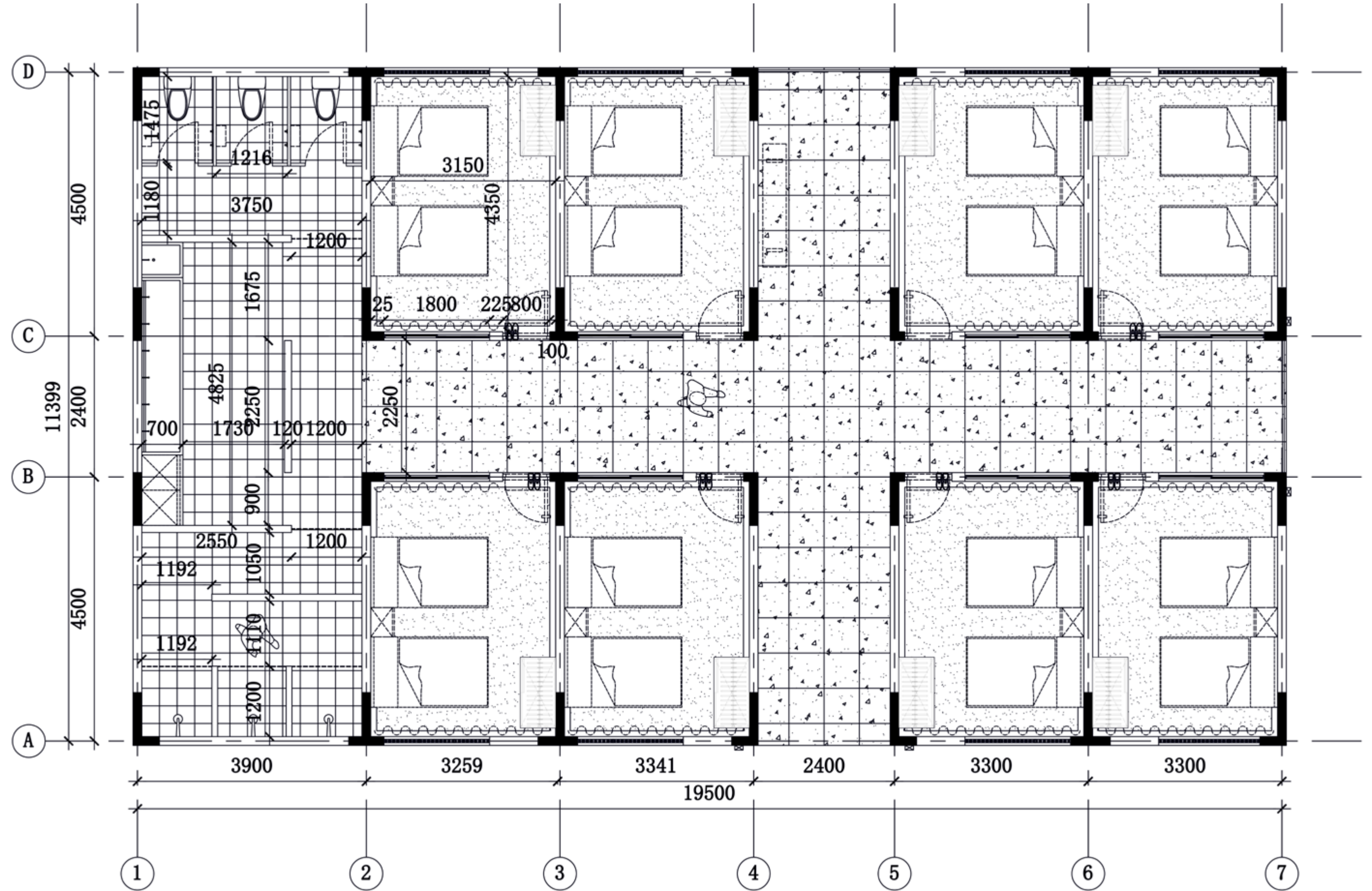
平面尺寸图
