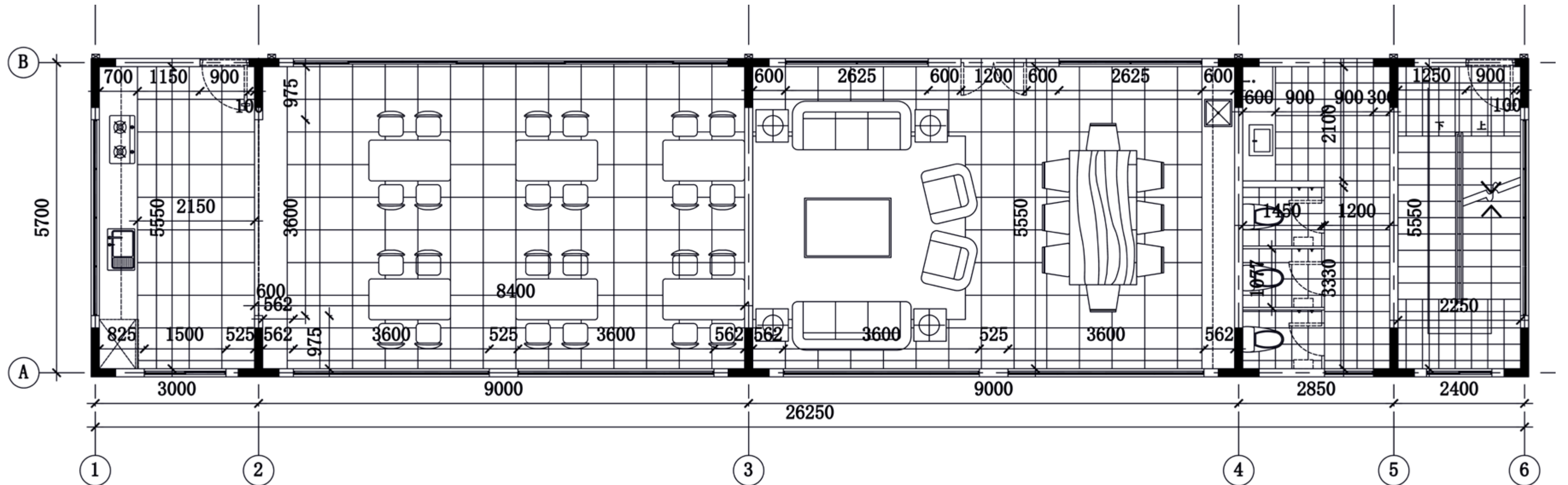
平面尺寸图
